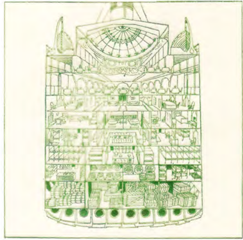
8. Coupe transversale d'un transatlantique
