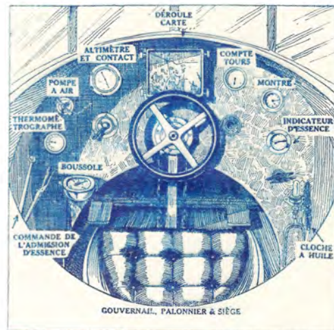
10. Siège du pilote et instruments de bord
