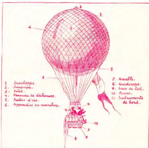
3. BALLONS LIBRES. - Un Sphérique
