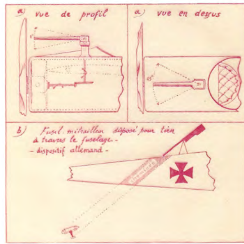
8. AVIONS DE GUERRE. - Dispositif des mitrailleuses (a) Tir à travers l'hélice. (b) Tir à travers le fuselage
